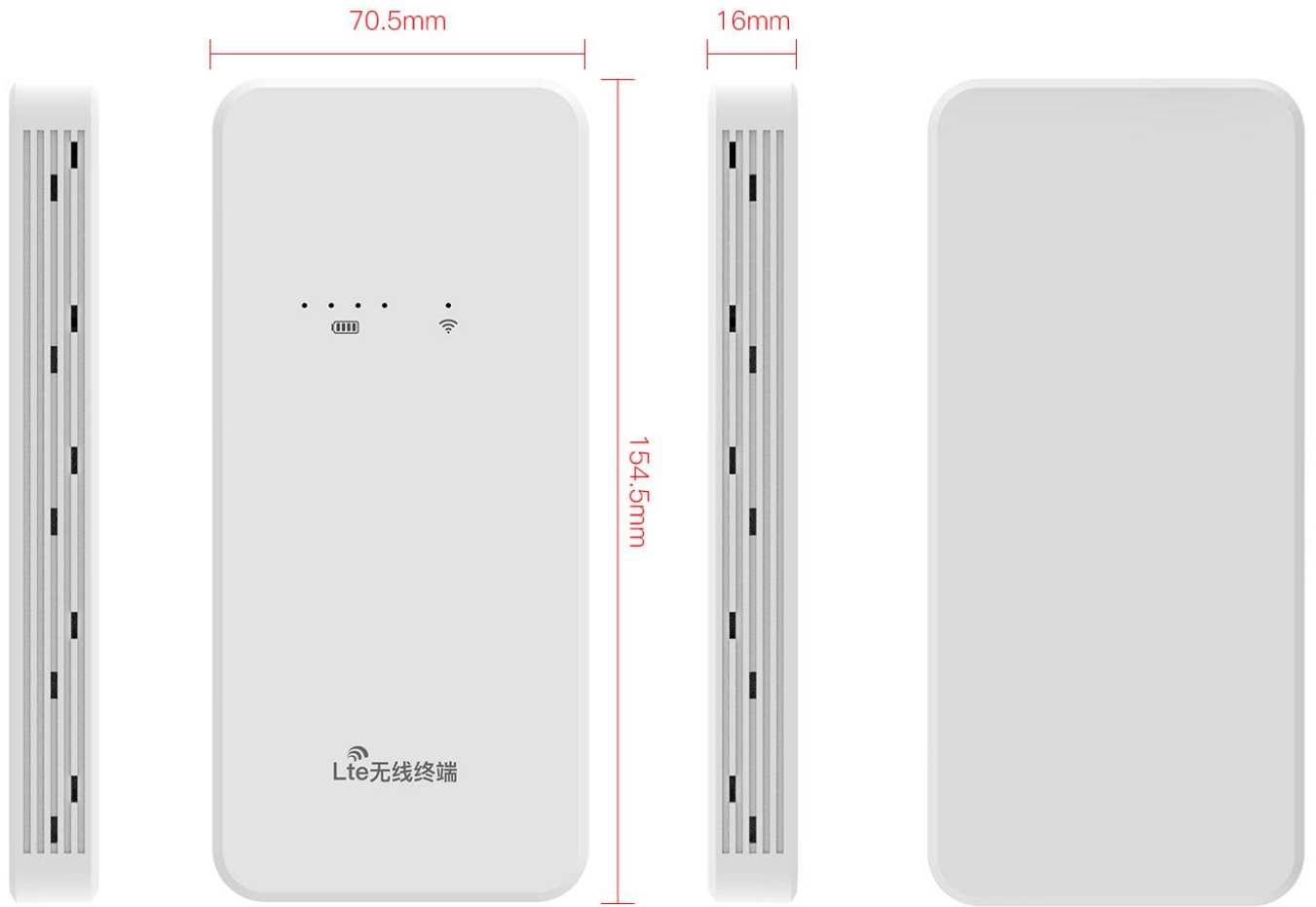
右视图
